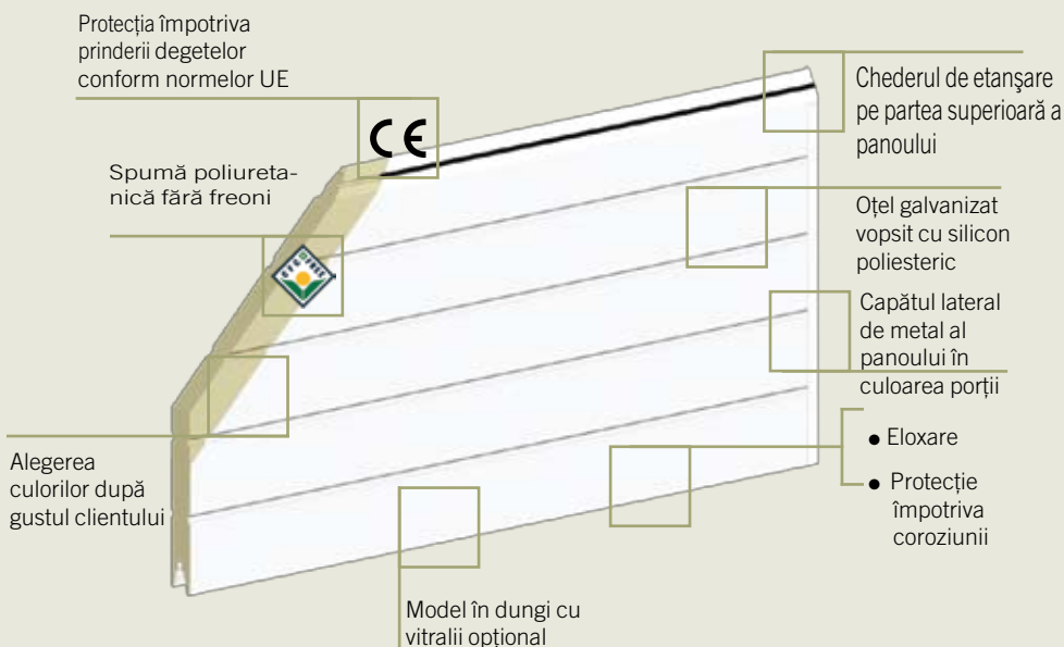
Poartă din oțel fără vitralii
